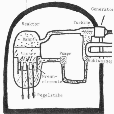
Siedewasserreaktor
