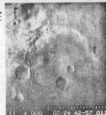
Marsoberfläche, am 14. 7. 1965 aus einer Höhe von 13 500 km mit Grünlinien durch Mariner 4 aufgenommen. Die wiedergegebene Fläche hat 240 km Kantenlänge. Sonnenlichteinfall unter 47° gegenüber dem Zenith von N (oben im Bild). Die runden Flächen sind also Vertiefungen (Krater).
