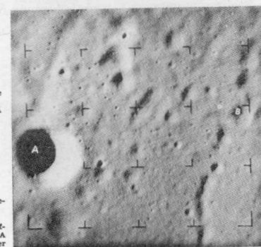
Marsoberfläche, am 14. 7. 1965 aus einer Höhe von 13 500 km mit Grünlinien durch Mariner 4 aufgenommen. Die wiedergegebene Fläche hat 240 km Kantenlänge. Sonnenlichteinfall unter 47° gegenüber dem Zenith von N (oben im Bild). Die runden Flächen sind also Vertiefungen (Krater).
