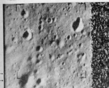
Abb. 3: Die letzte Aufnahme, die Ranger 9 aus 650 m Höhe machte. Die Kante des Bildes entspricht 73 m Länge. Aufsturztelle von Ranger 9 im weißen Kreis. Am unteren Rand, rechts von der Mitte (Pfeile), sind zwei Felsblöcke von etwa 1 m Durchmesser zu erkennen (Schatten rechts). Kleinste Details des Bildes etwa 50 cm.
