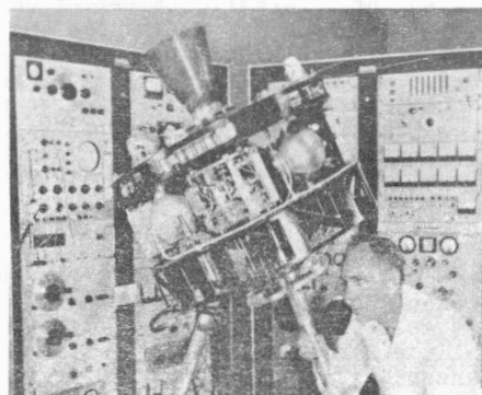
Dieses Bild zeigt den Syncom ohne seine Sonnenzellen. — This view shows Syncom without its solar cells.
