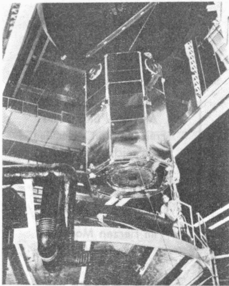
Zum längsten thermischen Vakuumtest über 1000 Stunden wird hier bei Grumman eine Zelle des Orbiting Astronomical Observatory in die große Weltraum-Prüfkammer eingebracht. Geprüft wird das passive Temperaturregelsystem des Satelliten. - A body of the Orbiting Astronomical Observatory being placed in the large space test chamber at Grumman, for thermal vacuum tests lasting more than 1,000 hours. In this particular experiment the satellite's passive temperature regulating system is to be tested. (Bild: Grumman)
